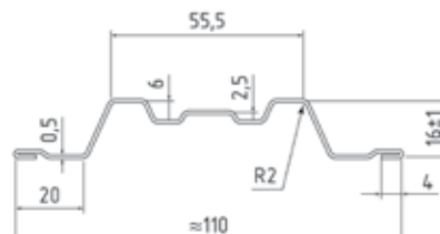
П-премиум
