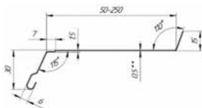
Отлив оконный
