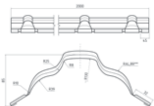
Конек PREMIUM
