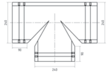
Тройник конька T-образный полукруглого
