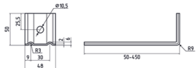
Кронштейн КР-50x2
