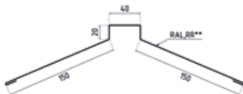
Конек фигурный
