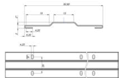
Планка усиливающая
