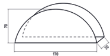
Заглушка конька полукруглого торцевая
