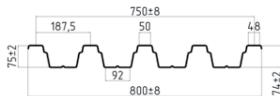
H-75
