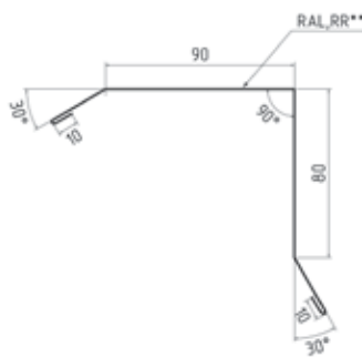
Ветровая (торцевая) планка
