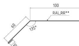
Капельник
