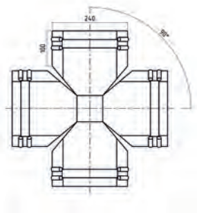
Четверник конька полукруглого
