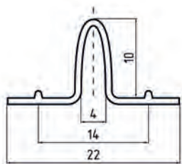
Маяк 0,6/1,0 мм
