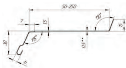
Отлив оконный
