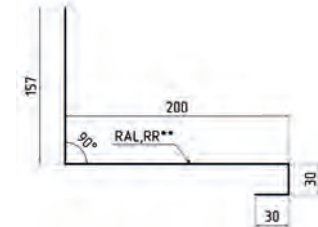
Планка примыкания нижняя к трубе
