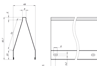
Ламель Duplex
