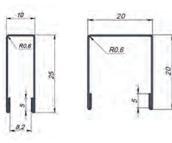
Планка П-образная для забора С-8/С-20/С-21
