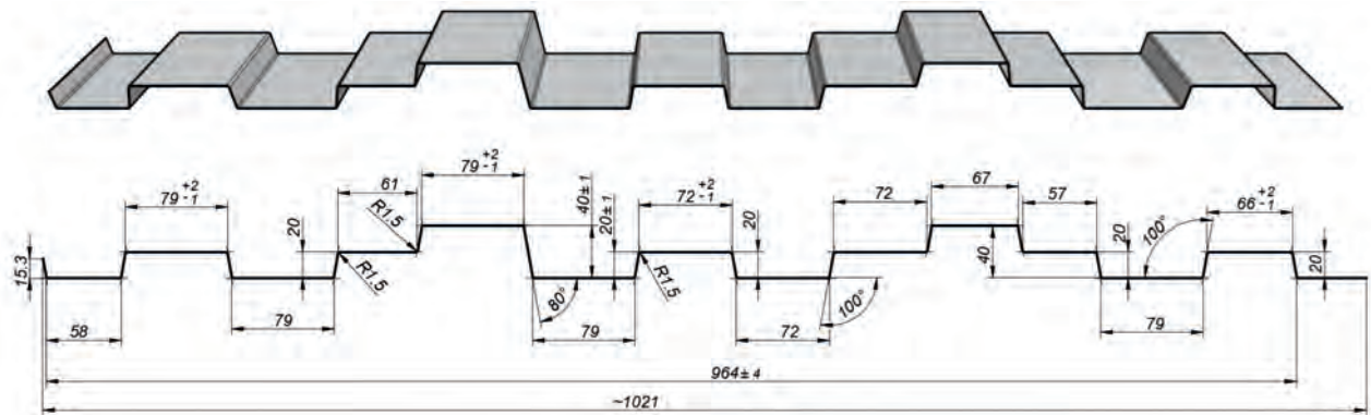
Панель BROOKLYN
