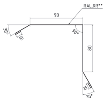
Ветровая (торцевая) планка
