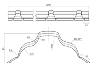
Конек PREMIUM
