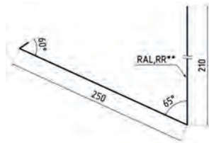
Планка примыкания верхняя к трубе
