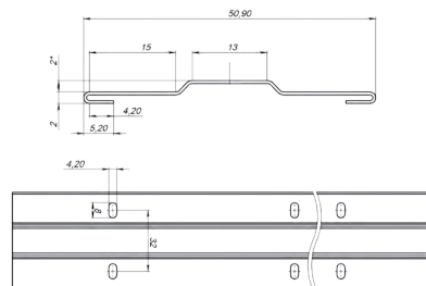
Планка усиливающая
