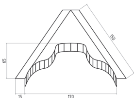
Заглушка конька конусная PREMIUM
