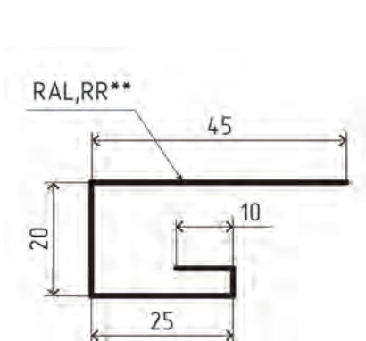
Планка завершающая (J-профиль)
