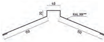
Конек фигурный
