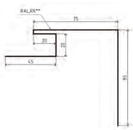
Откос
