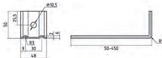
Кронштейн КР-50x2
