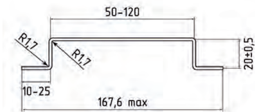
П-профиль
