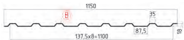
C-20 B
