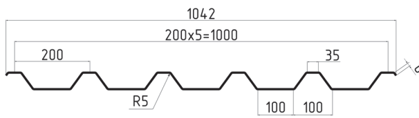
HC-44
