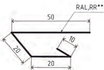
Планка стартово-финишная
