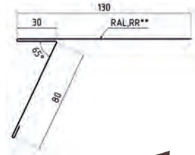
Планка карнизная
