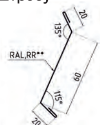
Планка примыкания в штробу
