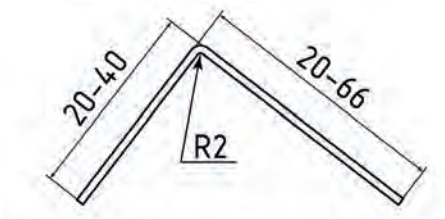
Г-профиль
